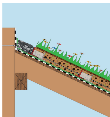
Schubsicherungssystem S
